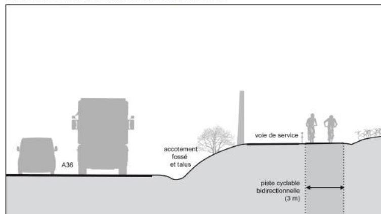
PROPOSITION D'AMÉNAGEMENT : PROFIL DE VOIE
